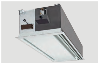
DCR-KPVS 天吊カセット形・1方向吹き出し形
